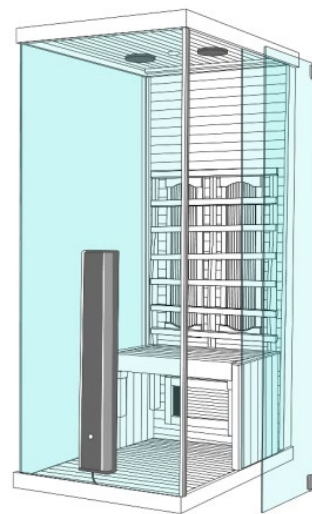
(10) Ansamblați balamalele
