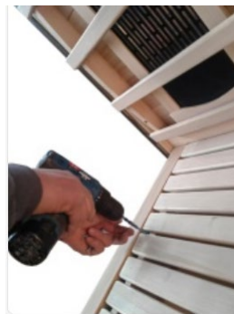
(9) Asamblați banca (șuruburi 4x50mm)
