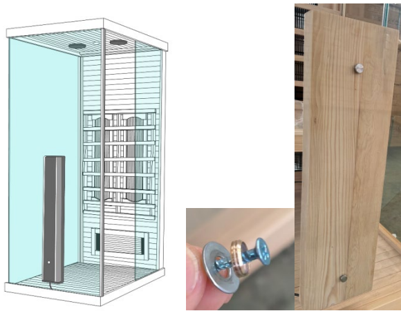
(7) Asamblați cutia de încălzire din față, Folosești șuruburi 4x20
