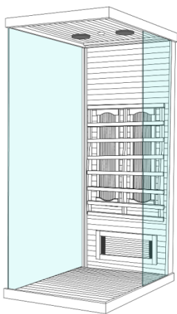
(5) Postavljeno streho in steklo pritrdite z vijaki
