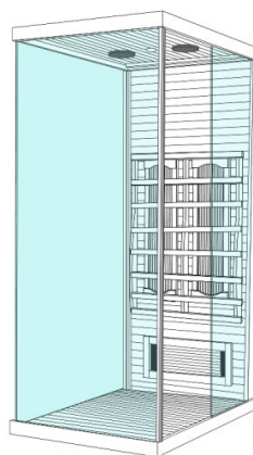
(6) Namestite sprednje steklo in uporabite vijake za steklo
