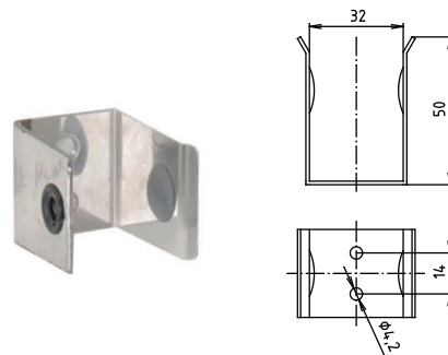
brzda / brake / Bremse:
